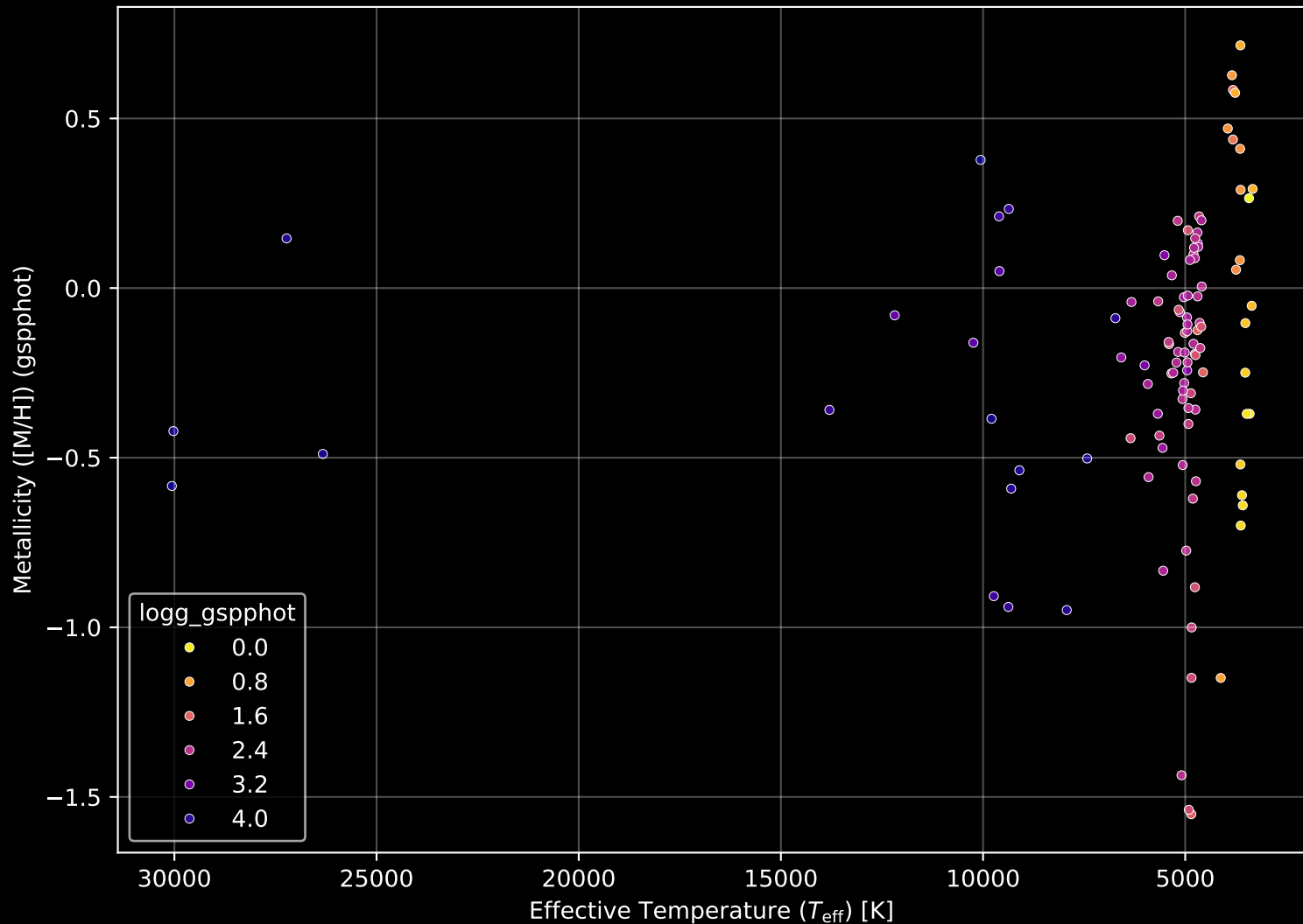
APOGEE DR17 Field: [357+05] Stellar Population Parameters (n= 110)
